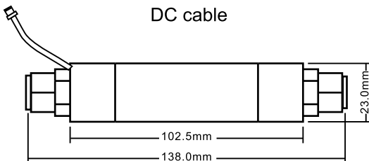
XHB254-2P cable
