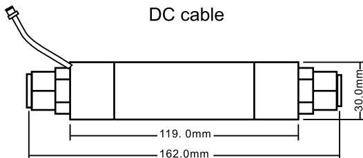
XHB254-2P cable
